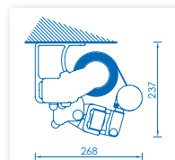
Asennus kattoon Ceiling installation
