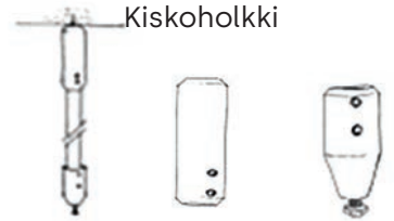
Kattotuen varsi 1000, 1500 tai 2000 mm Kattoholkki Kiskoholkki
